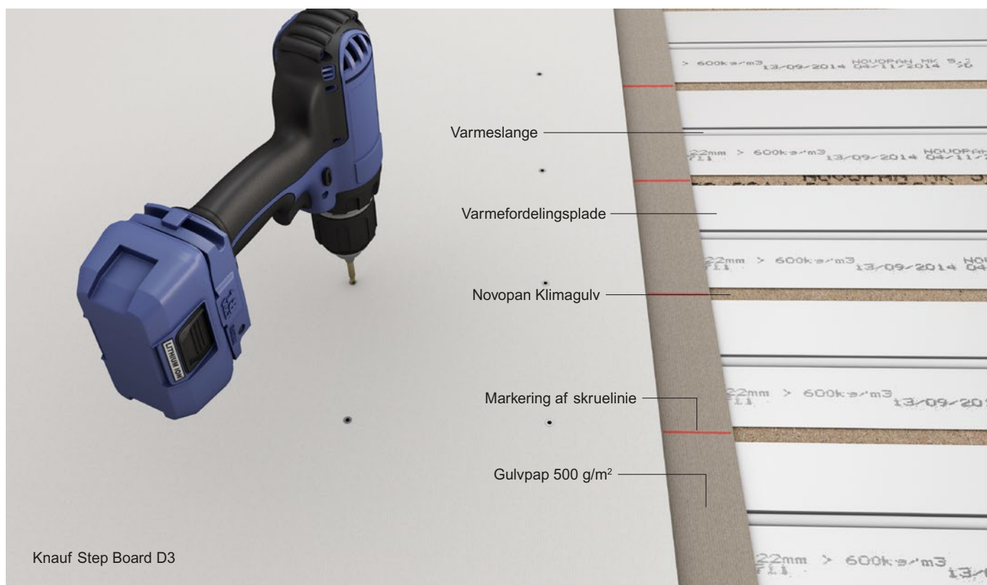
Figur 1 Novopan Klimagulv 22, 25 og 38 mm forstærket med Knauf Step Board som mellemlag under gulvbelægning, se side 2.
